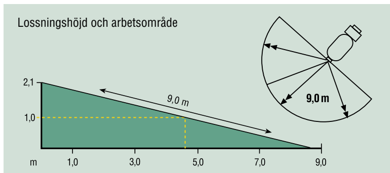
Räckvidder och lossningshöjder. Vid en lossningshöjd på t ex 1 meter är den maximala räckvidden ca 4,8 meter.
